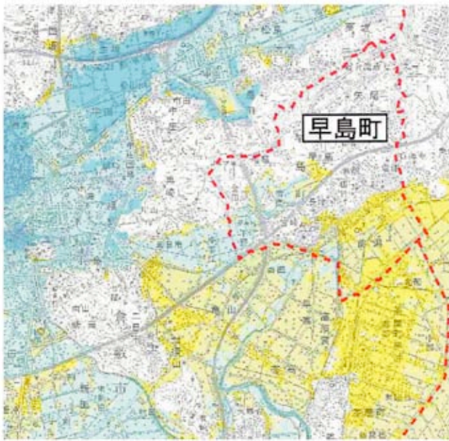
概ね150年に1回程度起こる大雨が降り、高梁川がはん濫した場合に想定される浸水の状況を、シミュレーションにより求めたものです。 出典：国土交通省岡山河川事務所ホームページから
